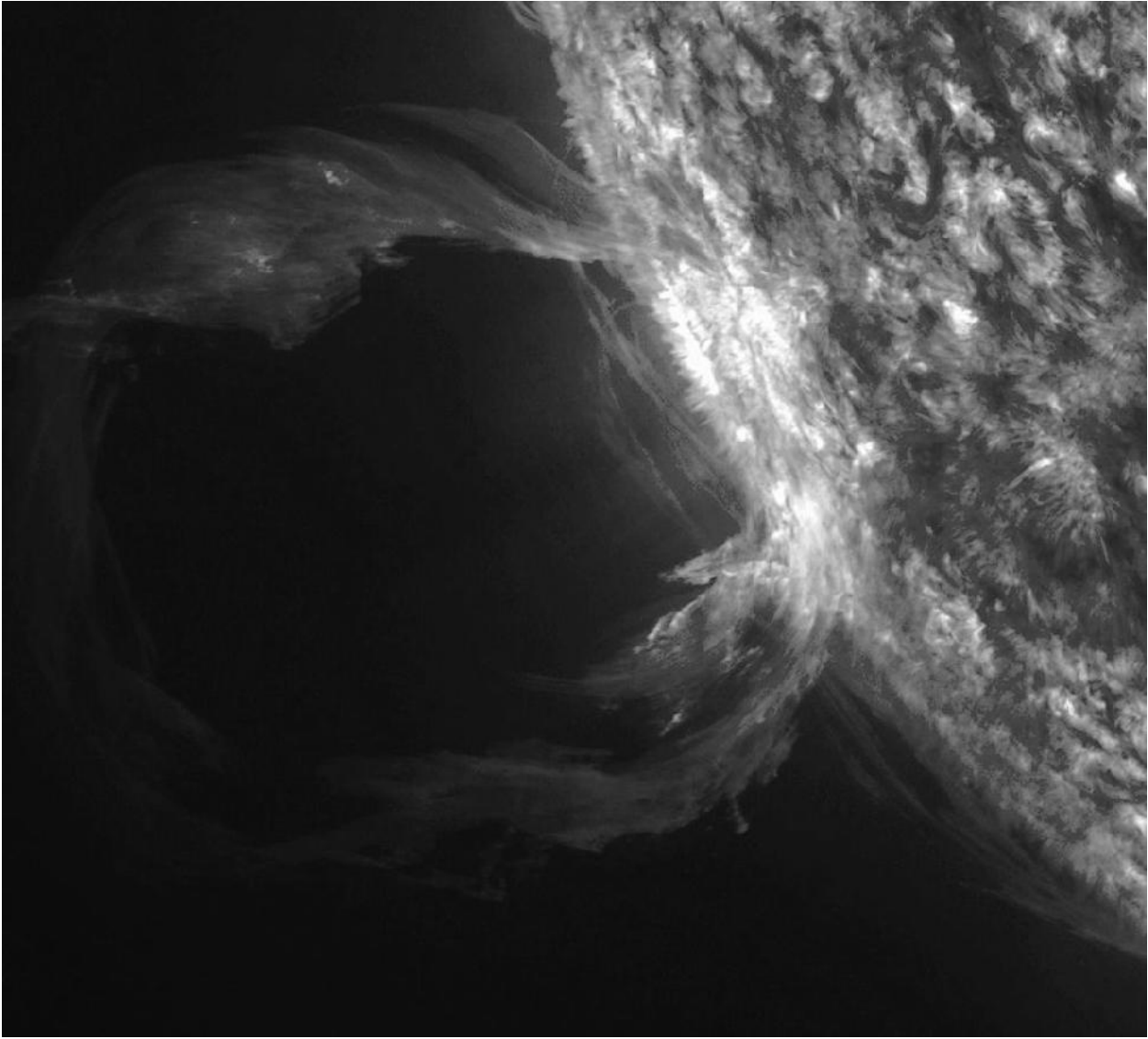
Llamarada solar
